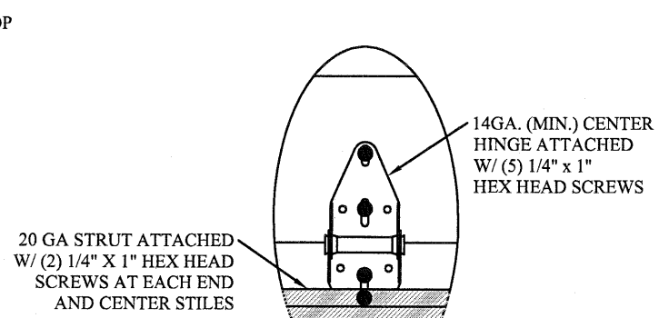
TYPICAL CENTER HINGE N.T.S. 2
