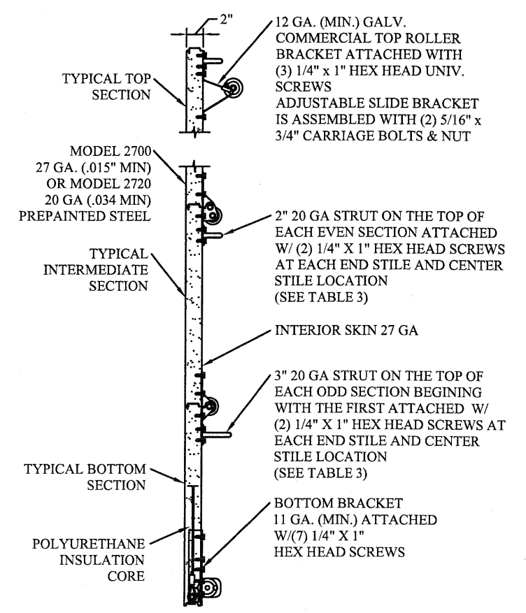
SECTION A-A (SIDE VIEW) N.T.S.
