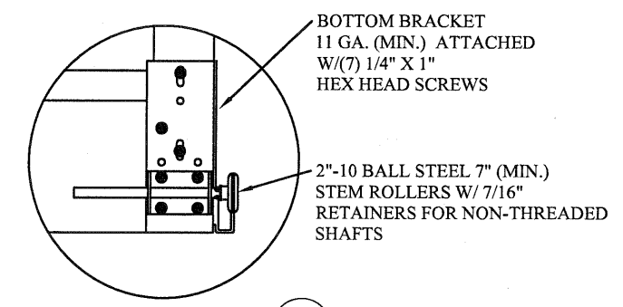
TYPICAL BOTTOM BRACKET N.T.S. 4
