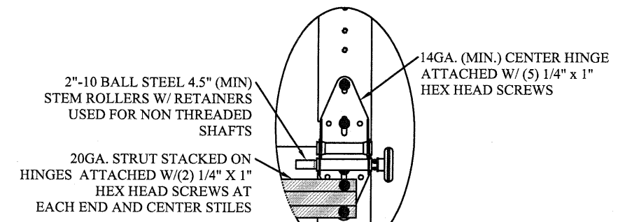
TYPICAL END HINGE N.T.S. 3
